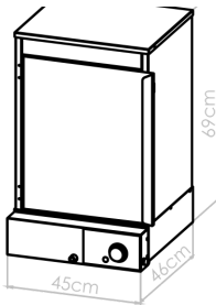
DIAGRAMA TÉCNICO · COTAS EN CM
