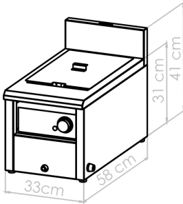
DIAGRAMA TÉCNICO · COTAS EN CM
