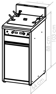
DIAGRAMA TÉCNICO · COTAS EN CM
