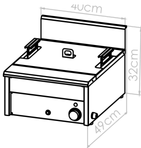
DIAGRAMA TÉCNICO · COTAS EN CM
