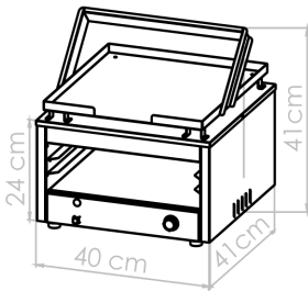
DIAGRAMA TÉCNICO · COTAS EN CM
