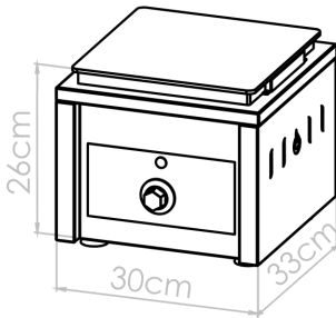
DIAGRAMA TÉCNICO · COTAS EN CM
