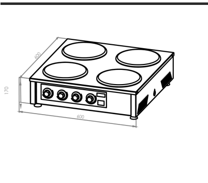
DIAGRAMA TÉCNICO · COTAS EN CM
