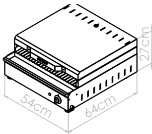
DIAGRAMA TÉCNICO · COTAS EN CM
